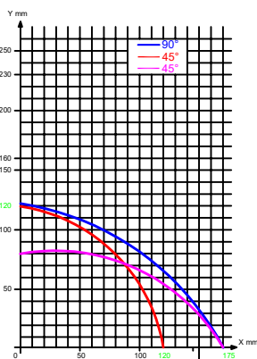
SSV - 16A/M
