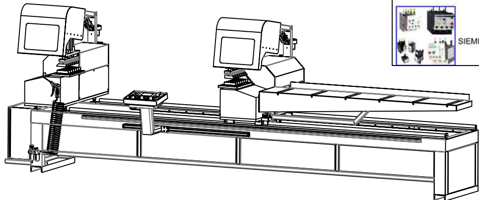
350/400 mm BLADE
