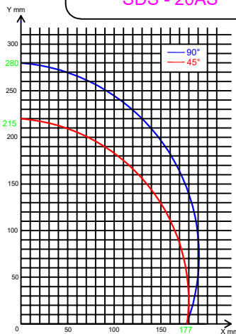
SDS - 20AS
