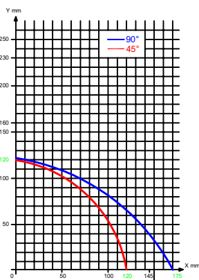
SSM - 16A/M
